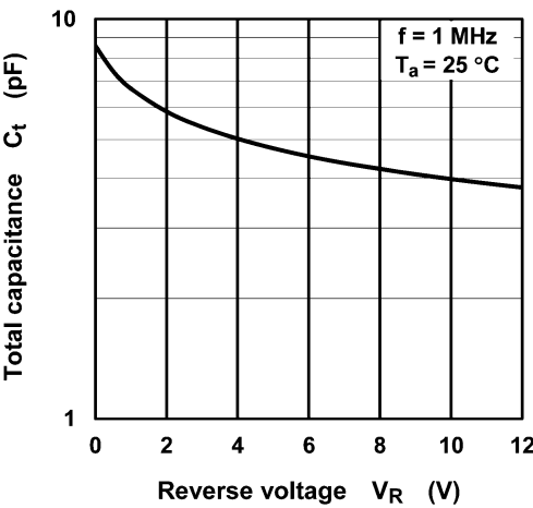
Fig. 9.3 C_t - V_R
