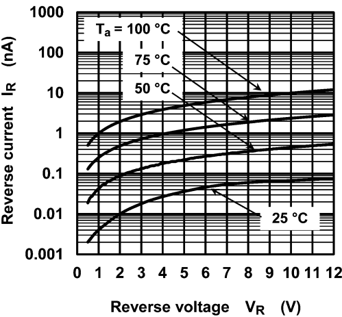
Fig. 9.2 I_R - V_R
