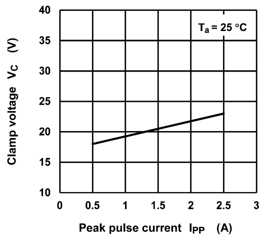
Fig. 10.1 V_C - I_{PP}
